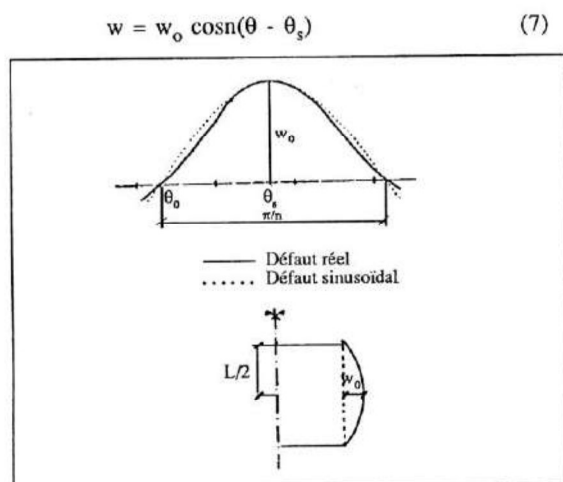
Figure 3 : Forme simplifiée du défaut.
