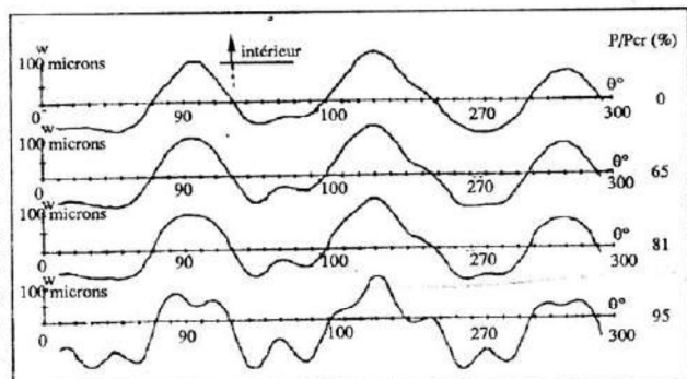
Figure 2 : Développement de la géométrie précritique sous pression externe, à mi-hauteur, d'une coque cylindrique quasi-parfaite.
