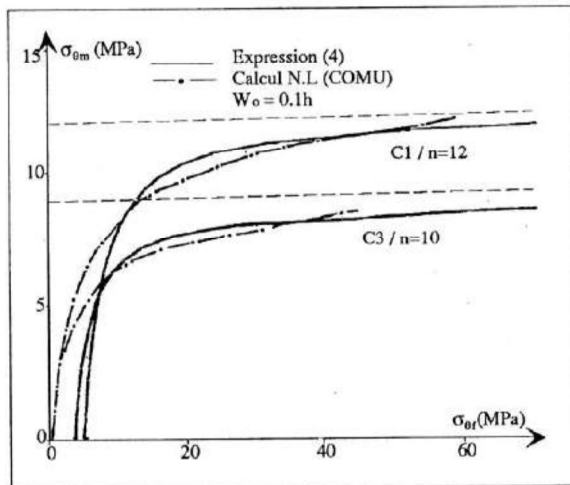
Figure 5 : Evolution des contraintes circonférentielles de flexion aux sommets des ondes à mi-hauteur.
